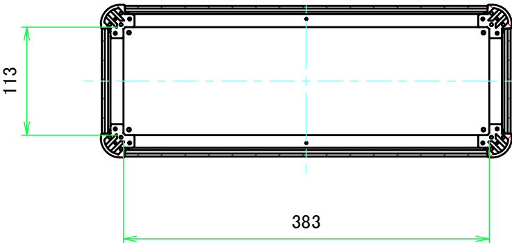
C-C ( 1 : 5.5 )
