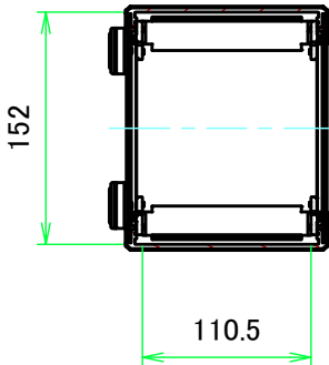
A-A ( 1 : 5.5 )
