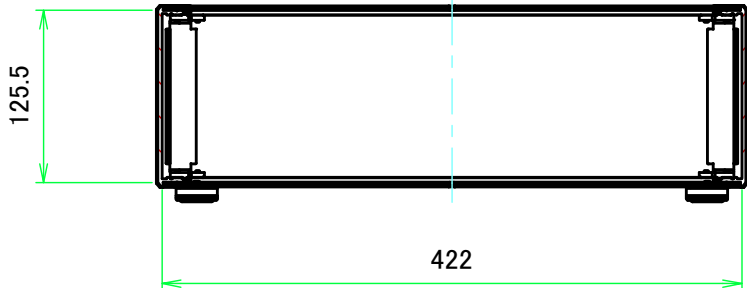
B-B ( 1 : 5.5 )
